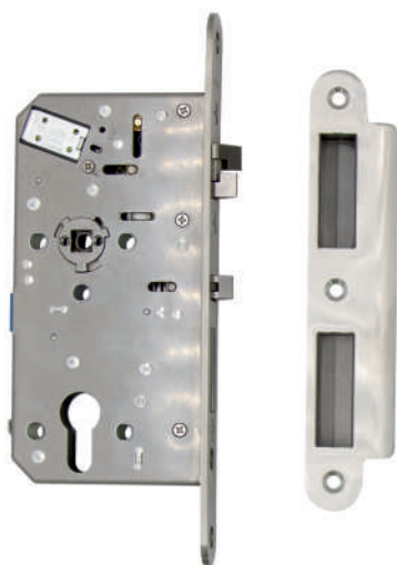
Электромеханический замок dktech DK551
